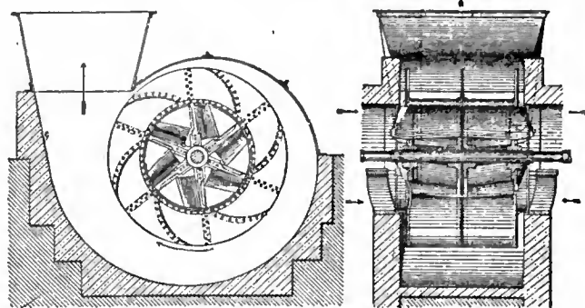
FIG. 19.—Capell Fan.
