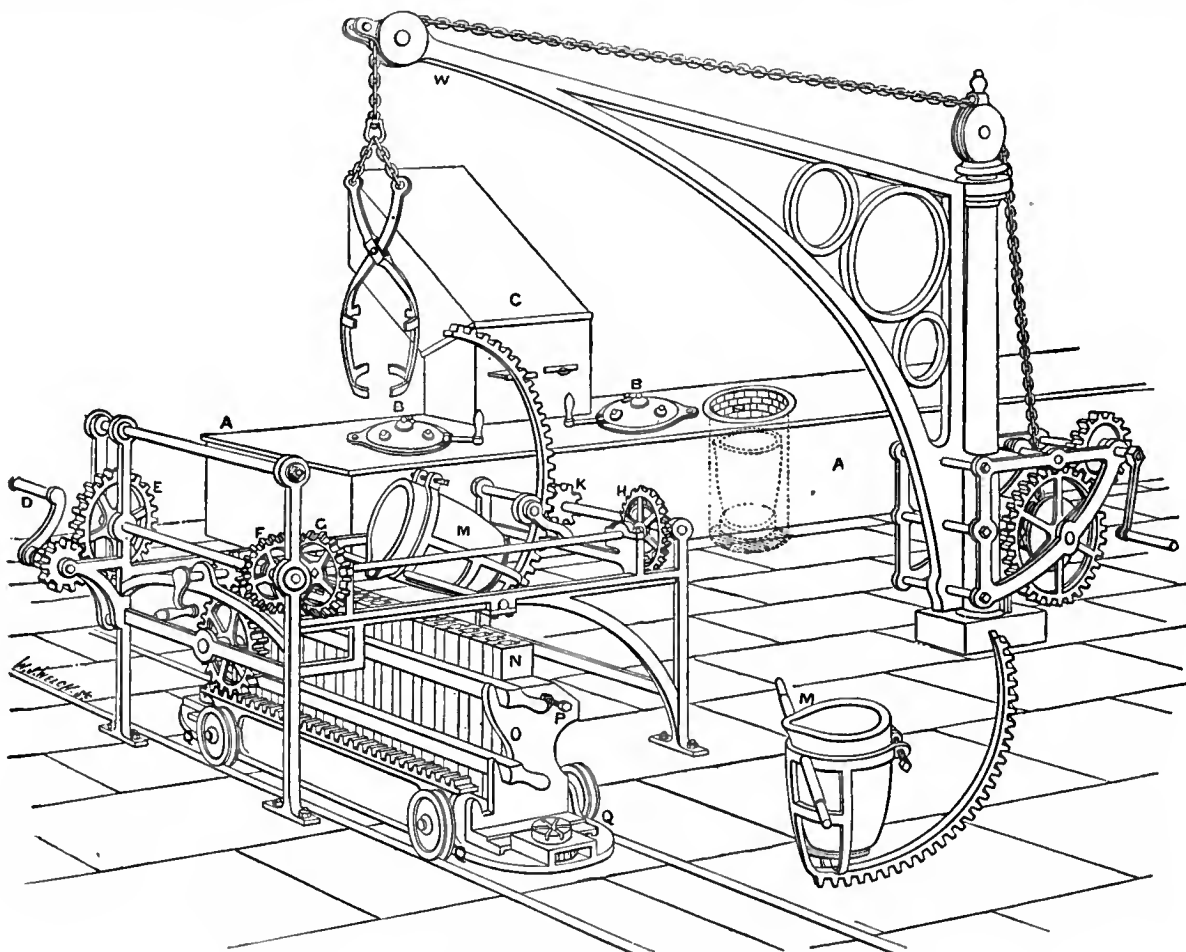
FIG. 1.—Furnace Apparatus.
